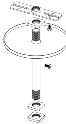
(Standard Pendant)
