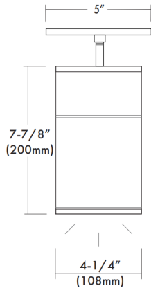
Pendant Mount
